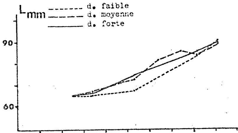
Fig. 4 : croissance linéaire du lot 2 capté en 1977
